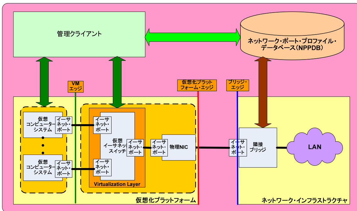
図 1 - 仮想化ネットワーク管理(VNM)モデル
