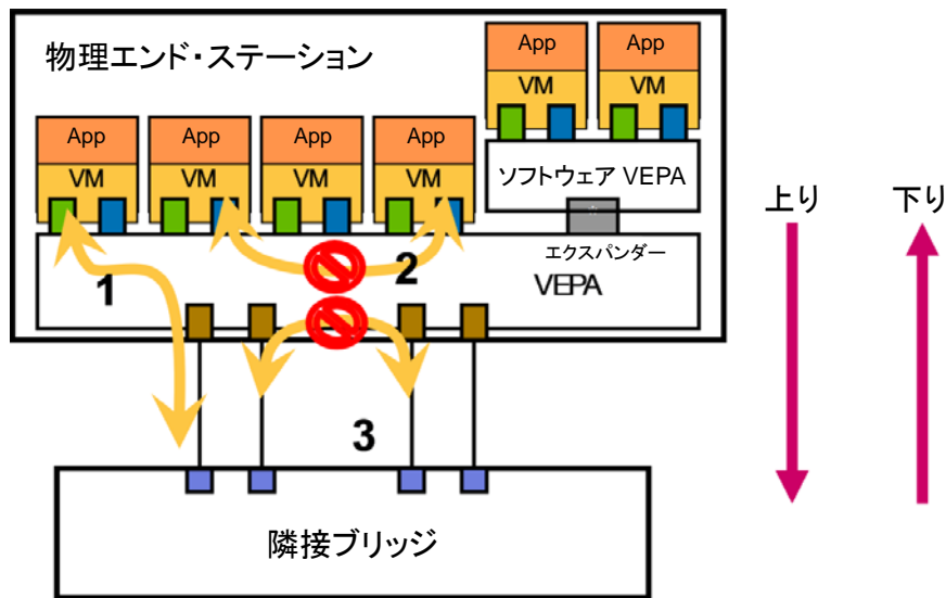
図 17 - VEPA フレームリレーのサポート
